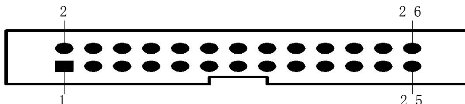
图 3-5 IDC26 针型并行接口插座引脚序号
