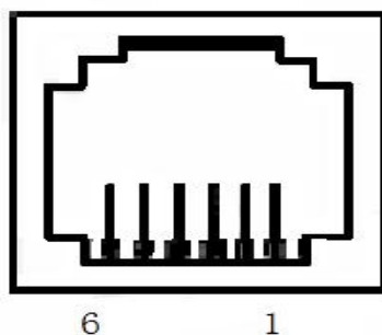
图 2-3 钱箱接口
