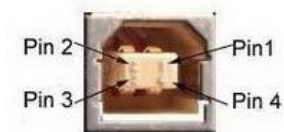
图 2-2 USB 接口
